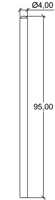
Eje timón varilla latón
