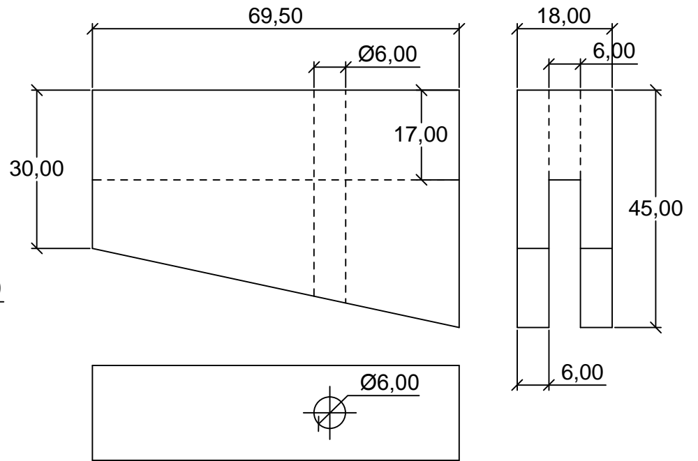
Pieza de refuerzo y centrado del timón
