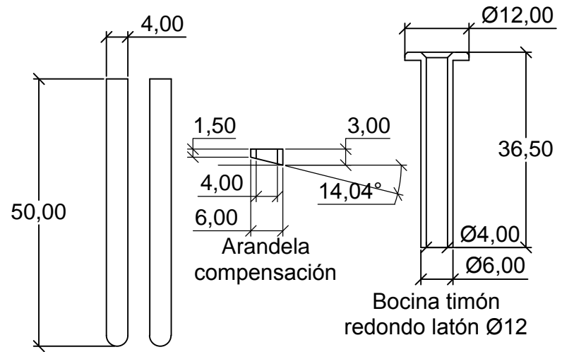
Tapas canal timón
